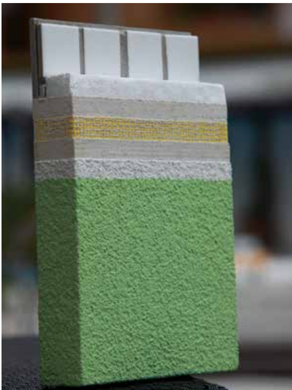
■飯店外牆翻新使用環保建材，此為解說樣品，最內層為舊磁磚，不同顏色代表由內而外的綠建材質。
